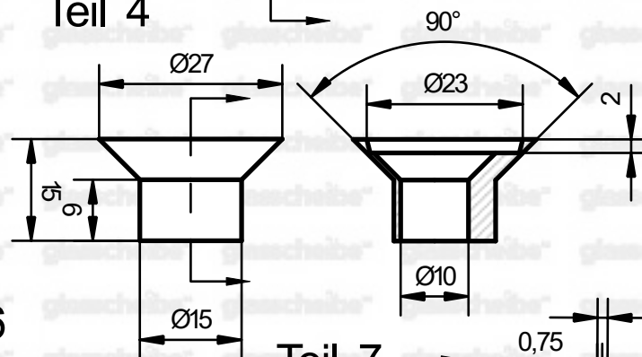
Schraube M6
